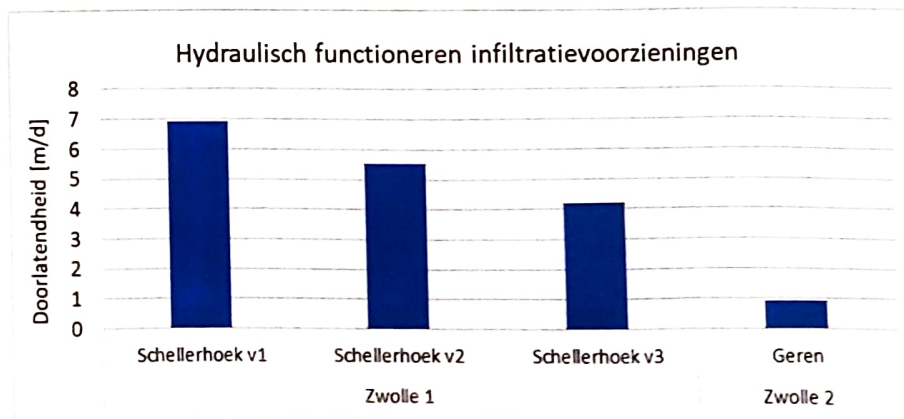
Infiltratiecapaciteiten proeven Zwolle v1 = vulling 1.
