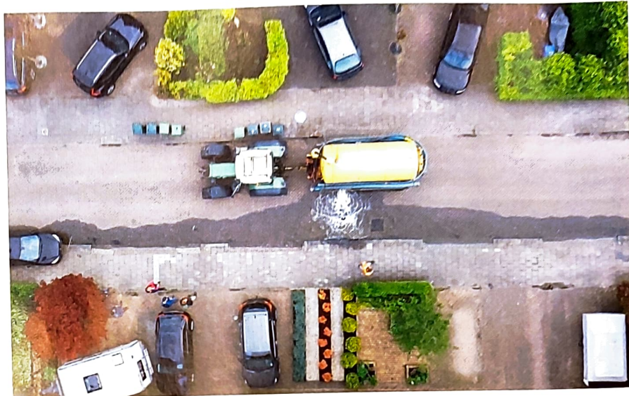
Full scale-test in Zuster van der Kolkstraat (Schellerhoek) Zwolle.
