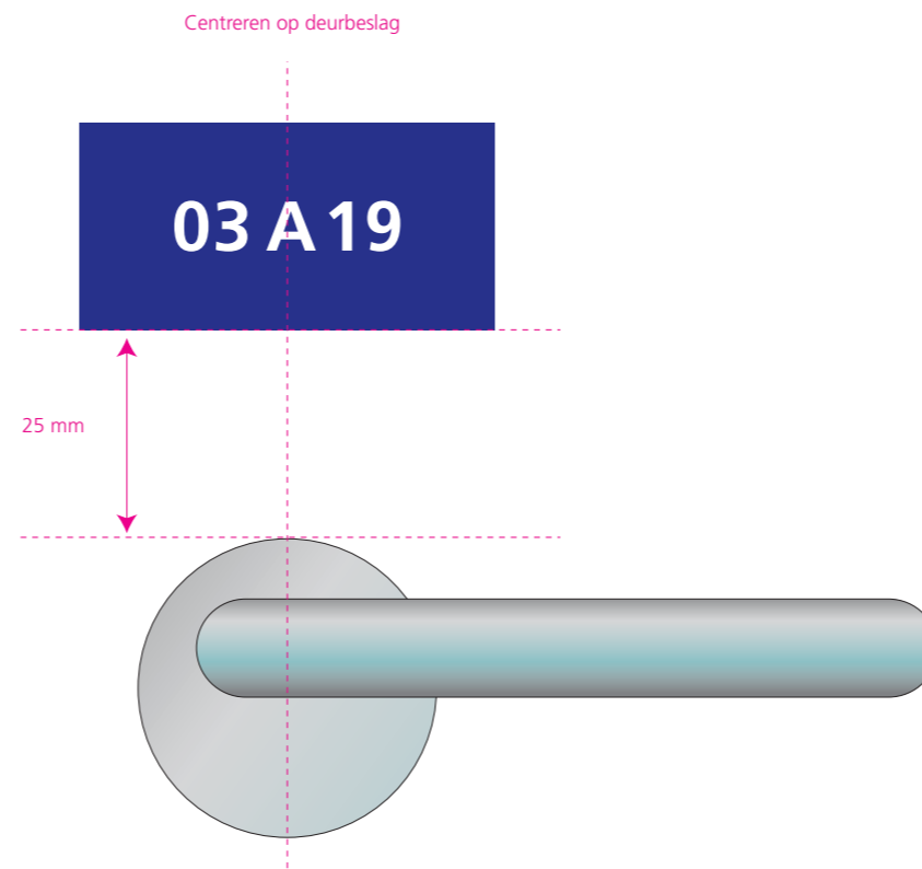
Positionering ruimtenummerplaatje
