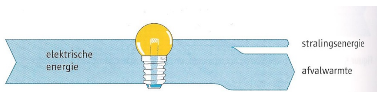
Figuur 12 Een iets andere systeemrepresentatie van Newton (versie vwo 2003, p178.)
