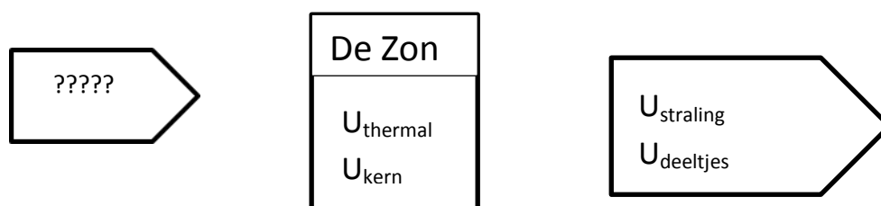
Figuur 11 Systeemdiagram van de zon
